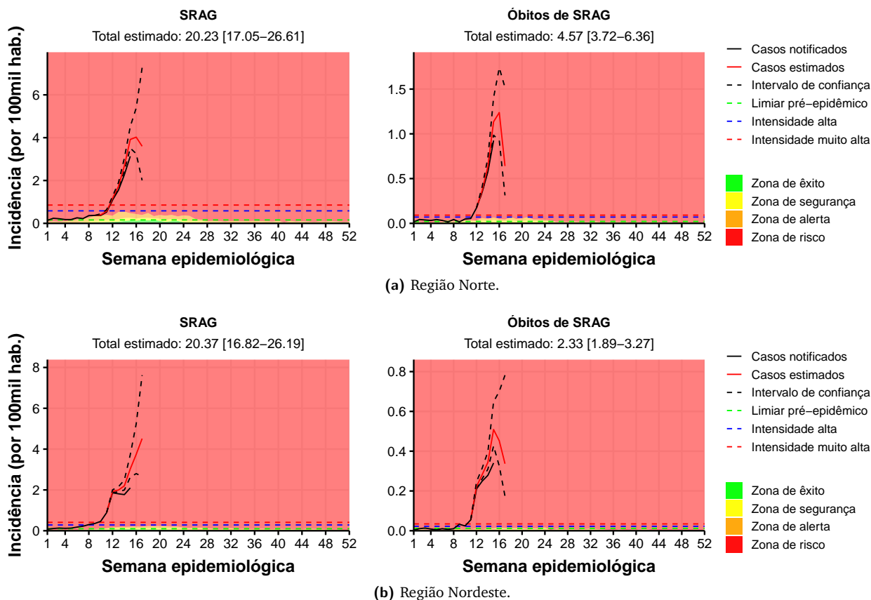
Figura 2. Séries temporais de síndrome respiratória aguda grave (SRAG) no país, por semana de primeiros sintomas. Casos (esquerda) e óbitos de SRAG (esquerda). As estimativa de casos recentes foi feita com base nos dados até a semana epidemiológica 17 de 2020.
